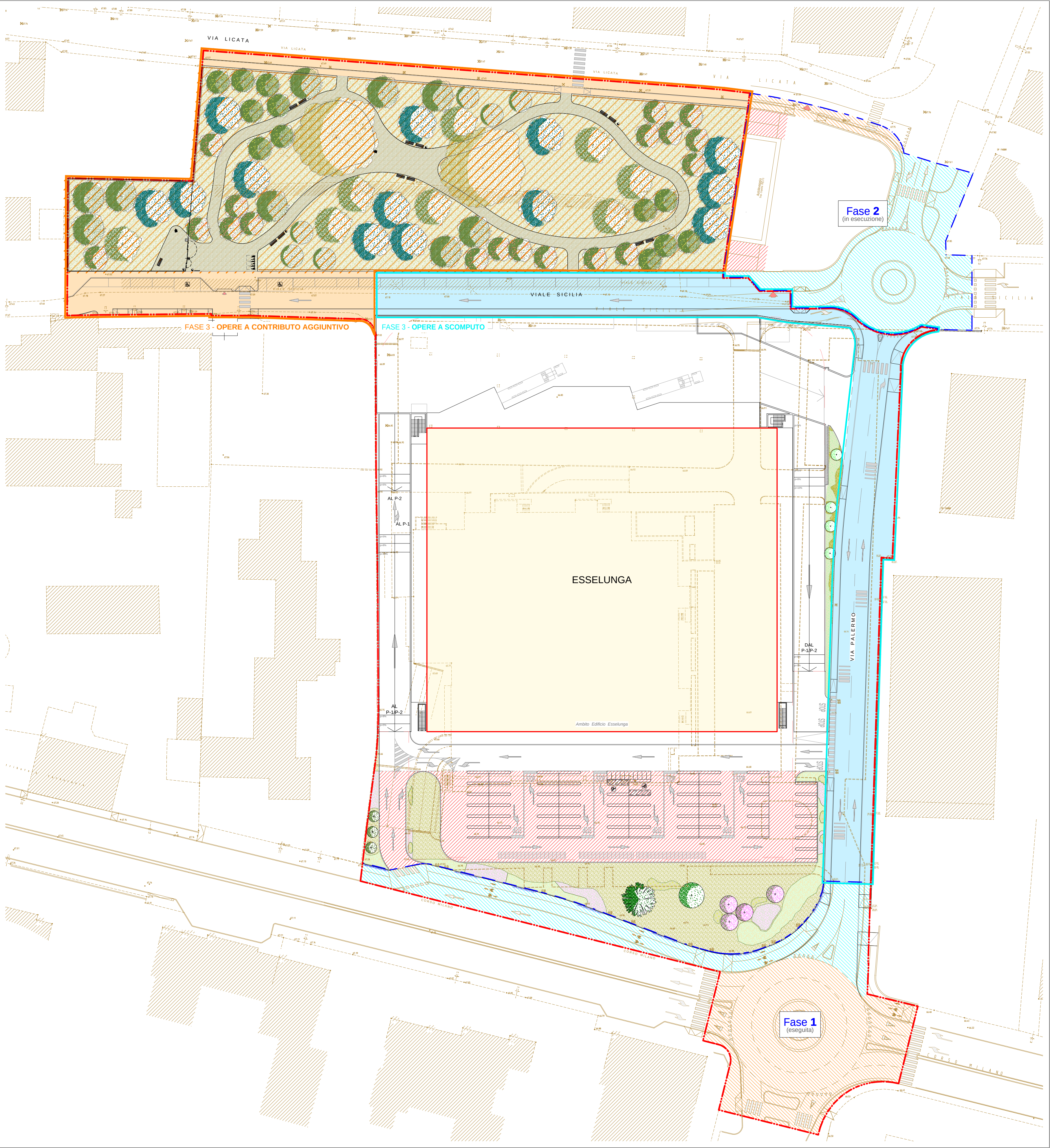
Planimetria generale del P.I.R.U.E.A. Esselunga 1:500
